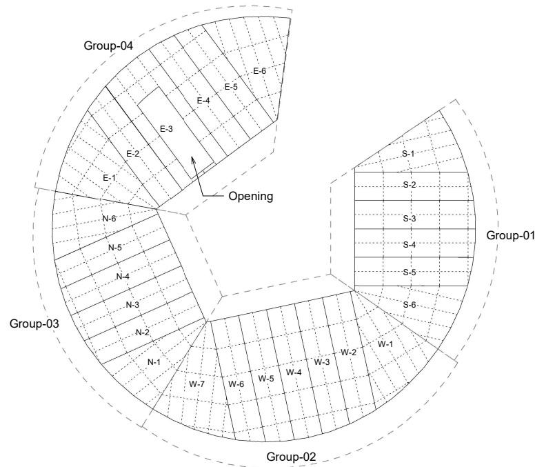
F1 Facade Flatten Sheet Detail
