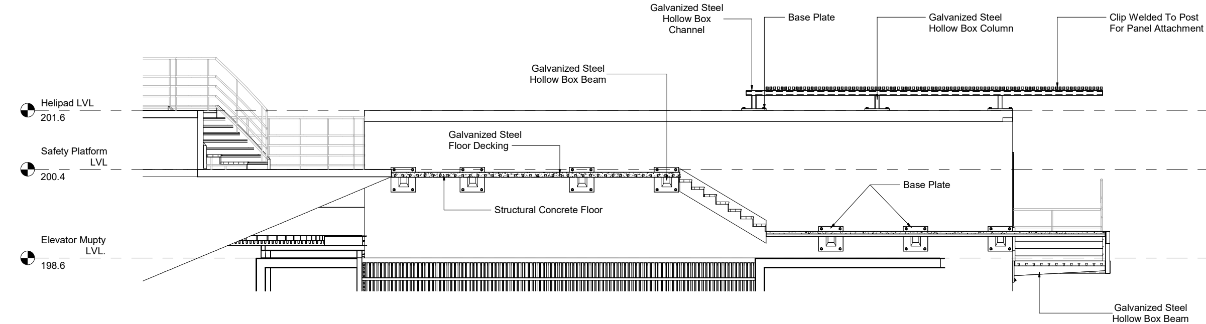
G1 Section 1A 1 : 35
